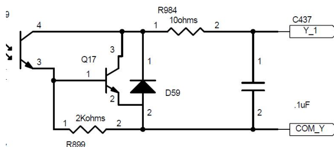
Grafika 12 Zasada działania wyjściowego suchego węzła
