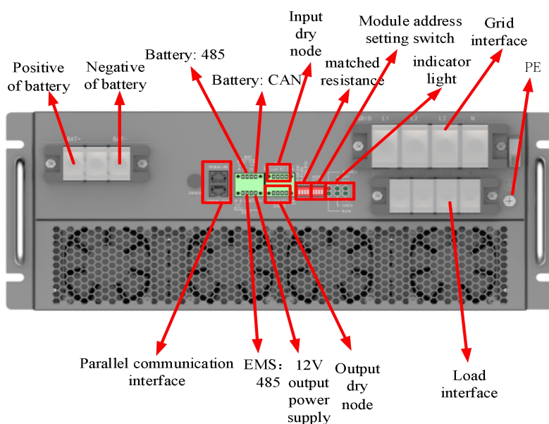
Grafika 10 Schemat definicji portu.
