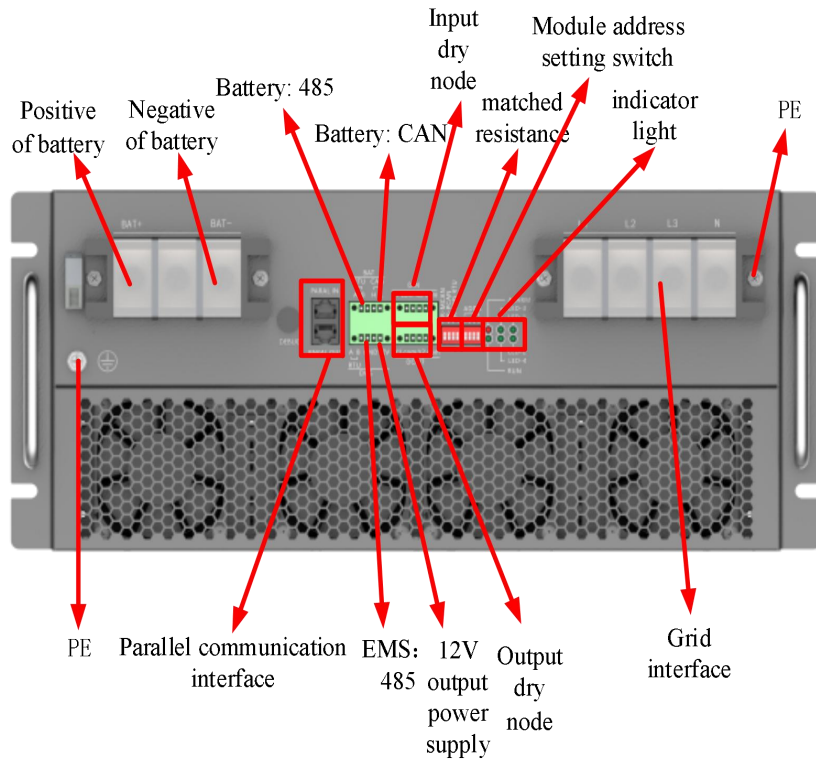
图 14 端口定义示意
