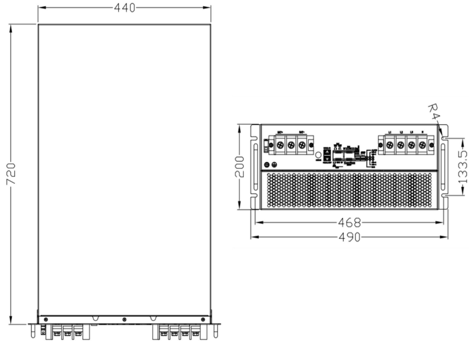
图 12 产品尺寸
