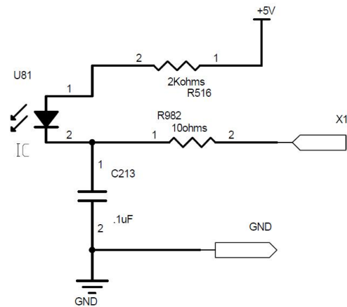
图 17 输入干节点内部原理图
