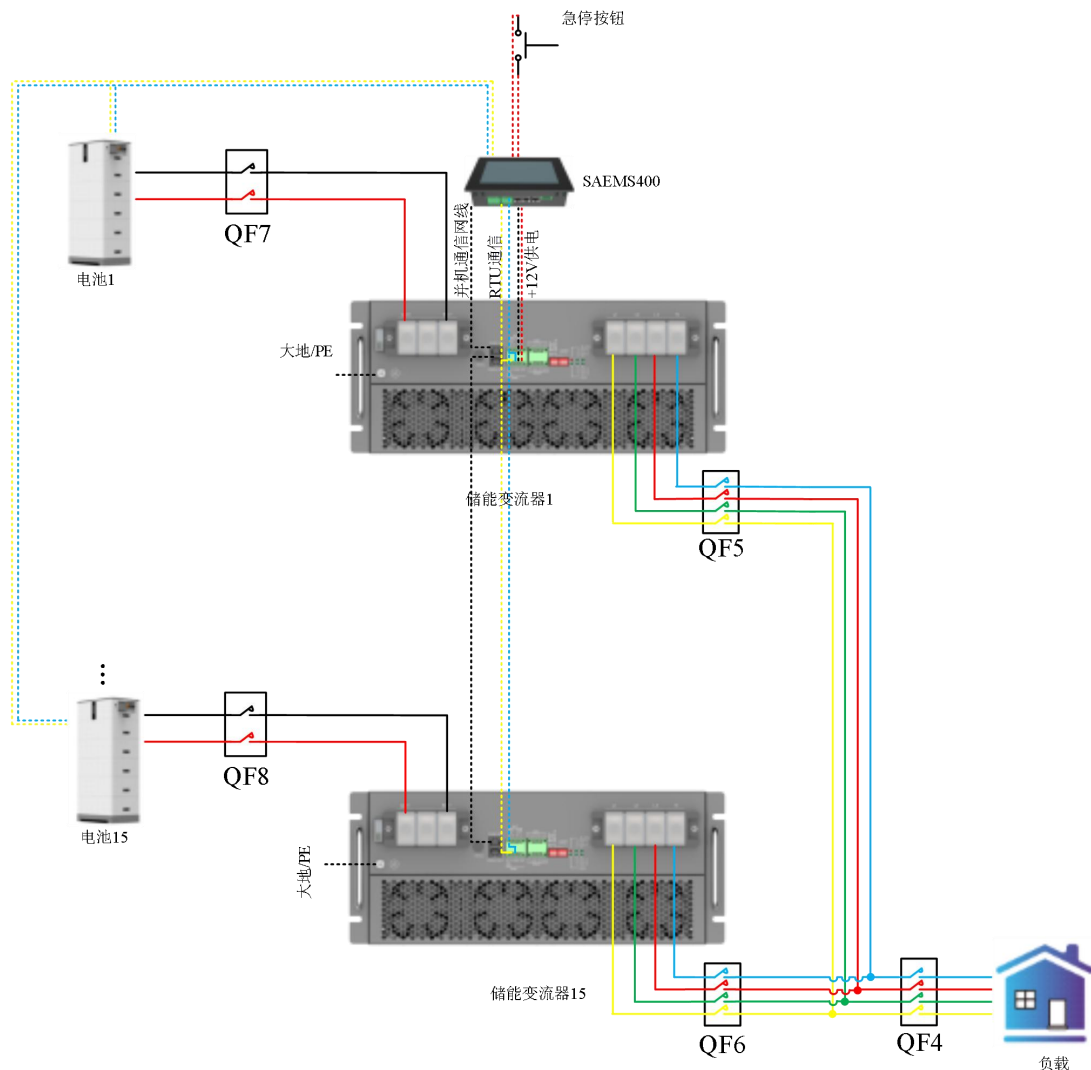
图 19 一簇一管理多机并联示接线意图
