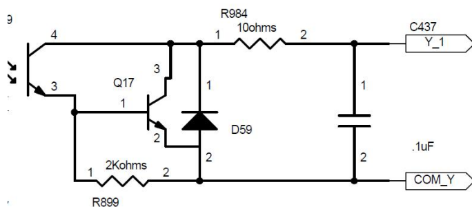
图 16 输出干节点内部原理
