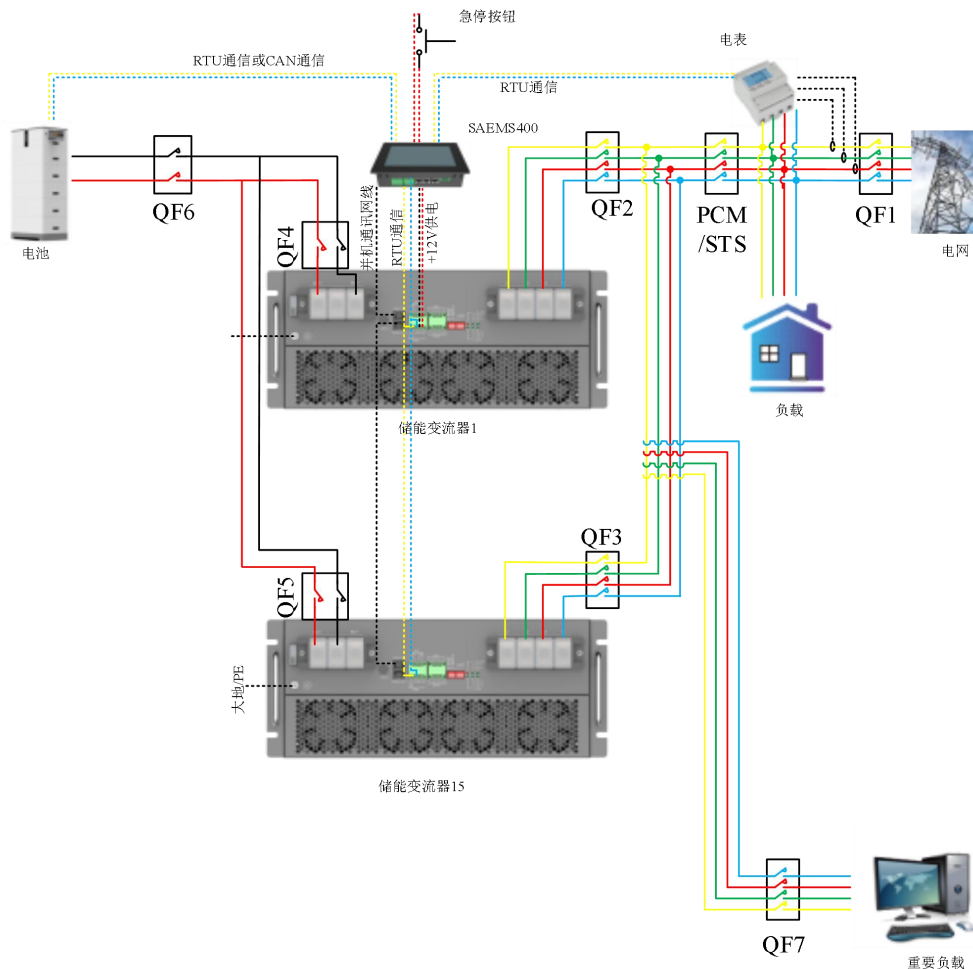
图 22 单电池包多机并联接线示意图
