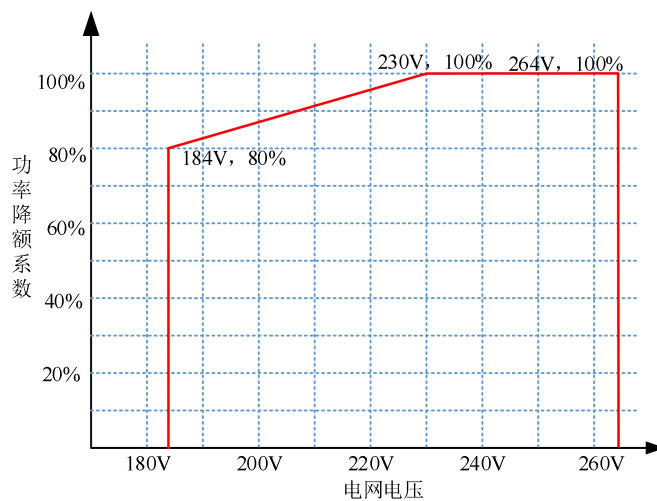
图 2 AC 充放电功率与电网电压关系
