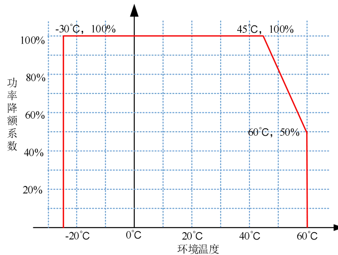
图 3 AC 充放电功率与环境温度关系
