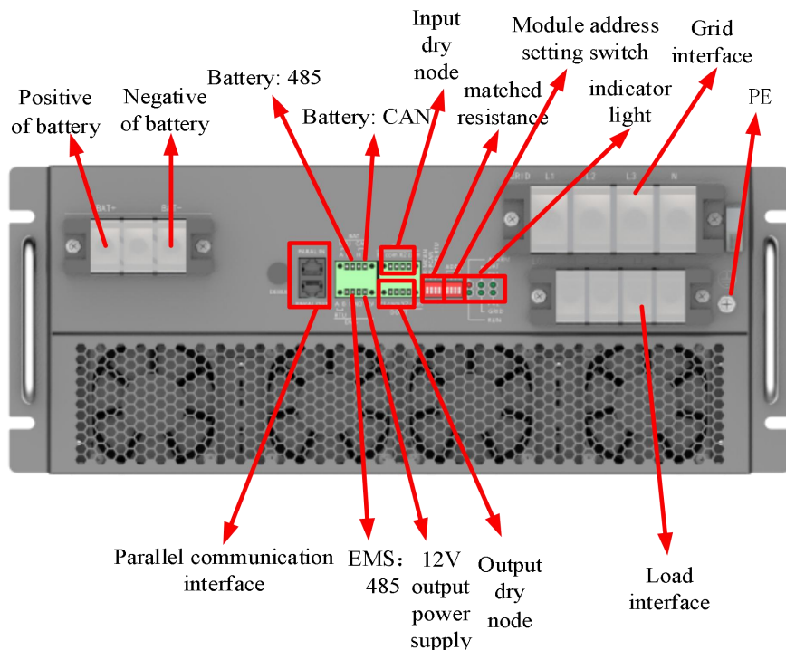
图 10 端口定义示意图
